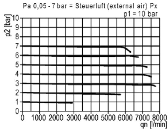
KMRZ 流量曲線圖
